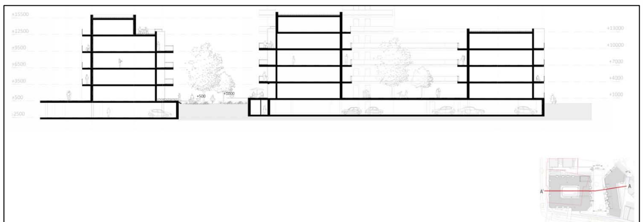
Figuur 2. Dwarsdoorsneden van de beoogde nieuwe situatie. Het vloerniveau van de kelderverdieping ligt 2,5 meter beneden maaiveld. Tekening d.d. 14 februari 2025 (Bron: Aangeleverd door de opdrachtgever).
