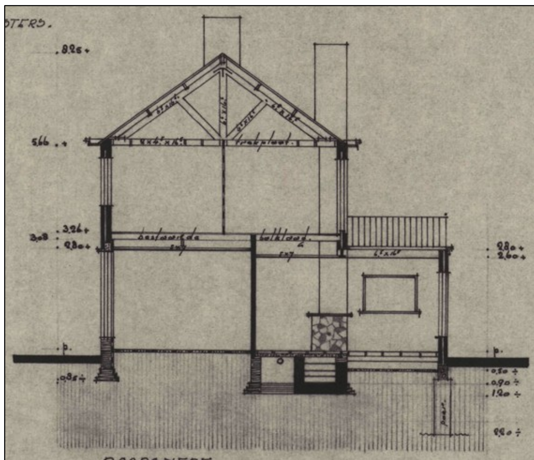
Figuur 8. Doorsnede van het huis met adres Mierloseweg 22.
